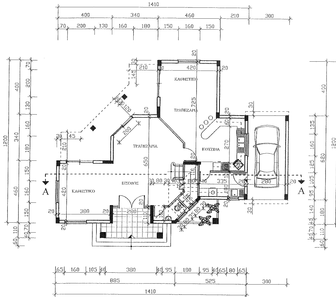
ΚΑΤΟΨΗ ΙΣΟΓΕΙΟΥ
