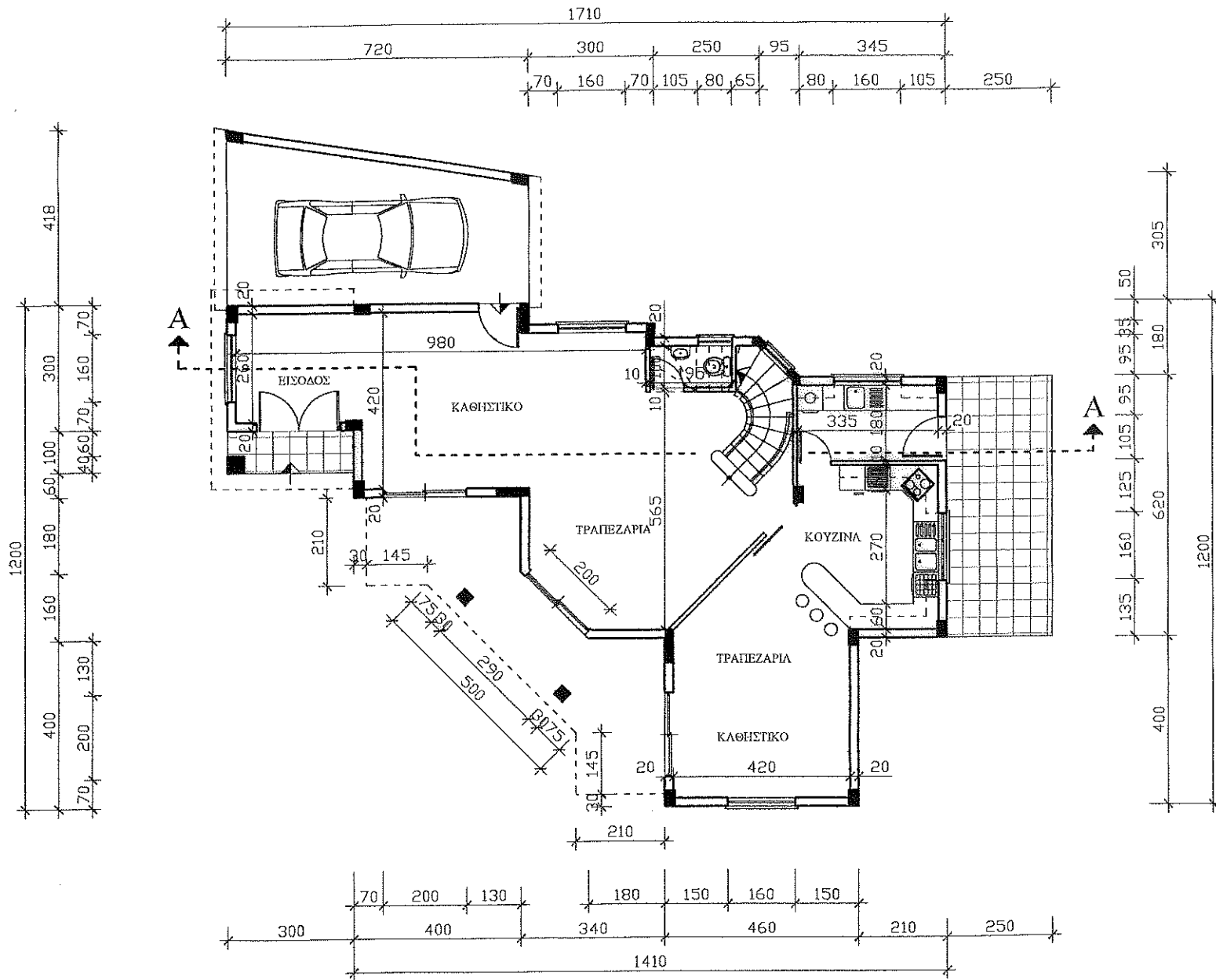
ΚΑΤΟΨΗ ΙΣΟΓΕΙΟΥ
