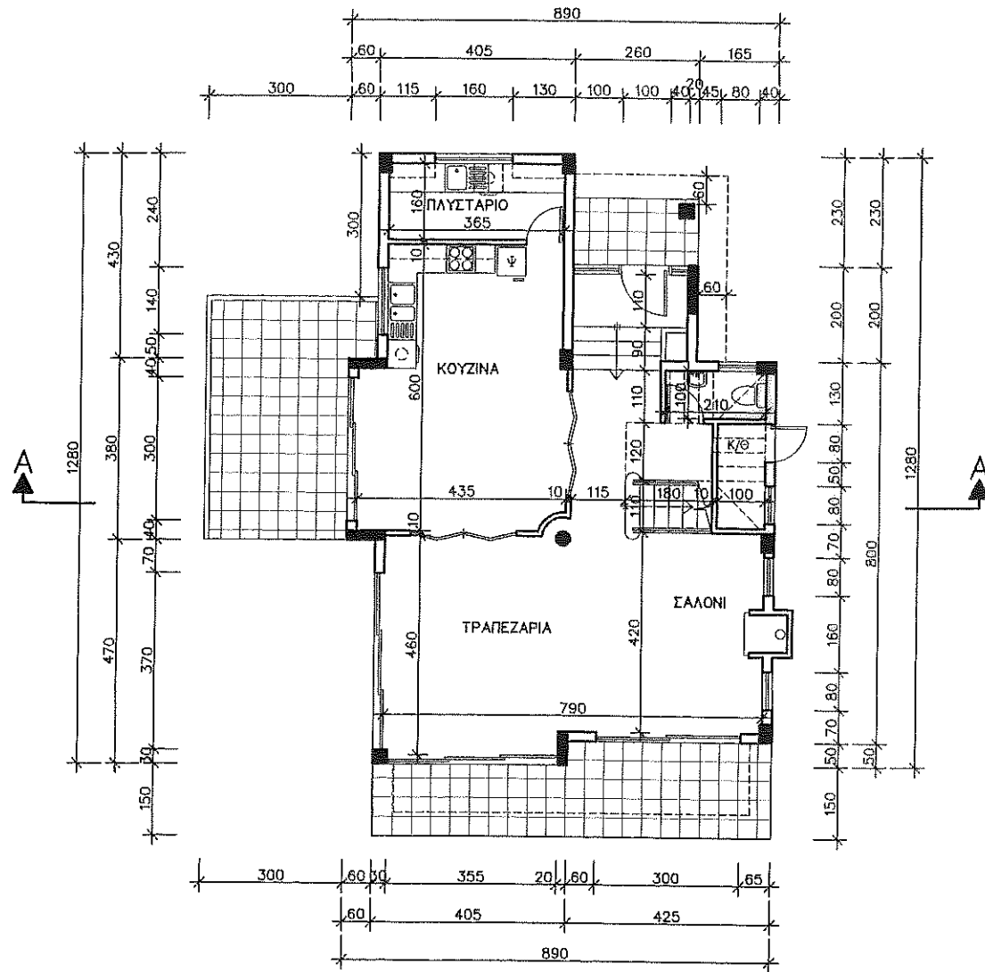
ΚΑΤΟΨΗ ΙΣΟΓΕΙΟΥ
