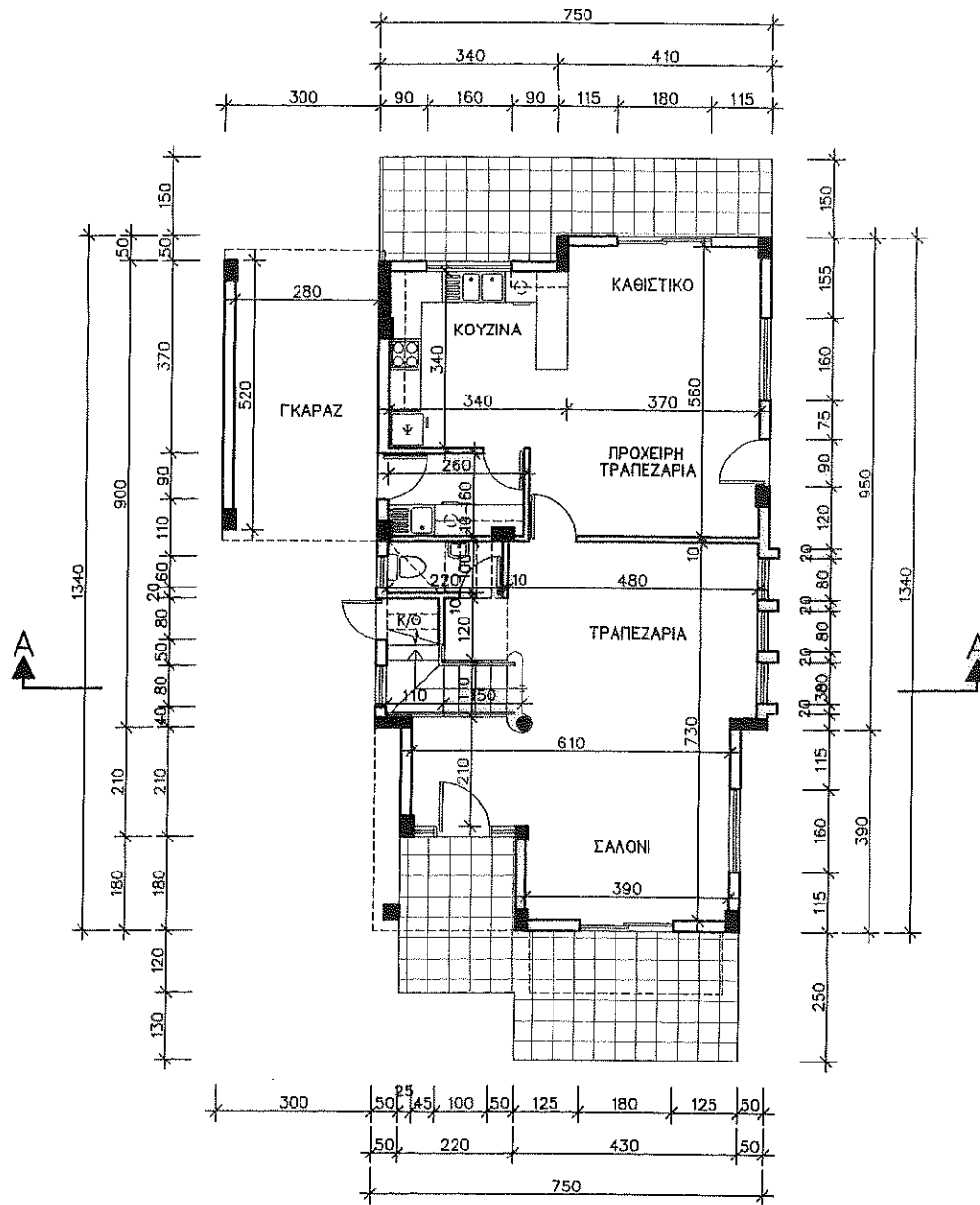
ΚΑΤΟΨΗ ΙΣΟΓΕΙΟΥ
