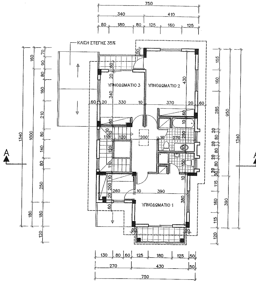
ΚΑΤΟΨΗ ΟΡΟΦΟΥ
